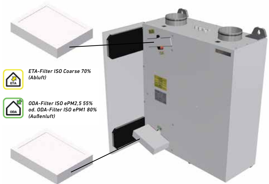
LG 150 mit geöffneter Fronttür für Filterwechsel, (einfaches Öffnen durch Aufschrauben der Schnellverschlüsse)
