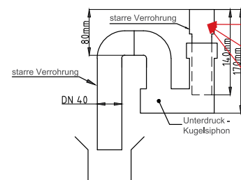
Beispiel: Kondensatanschluss mit Anbauerschraubungsstück und Kugelsiphon HL 136.3
