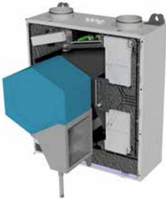
Kondensat-Tasse mit Kondensat-Anschluss R 1/2" AG
